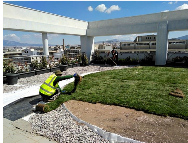
Εγκατάσταση και κατασκευή πράσινου δώματος των κτηρίων Εθνικής Τράπεζας
